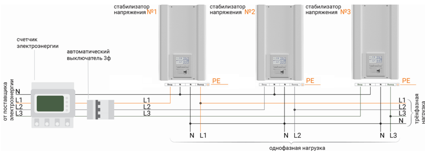
Рисунок 4. Схема подключения стабилизатора к трёхфазной сети
