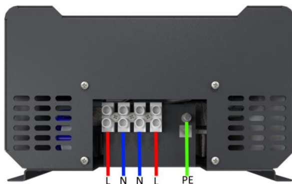
Рисунок 2. Схема подключения к клеммной колодке стабилизатора
