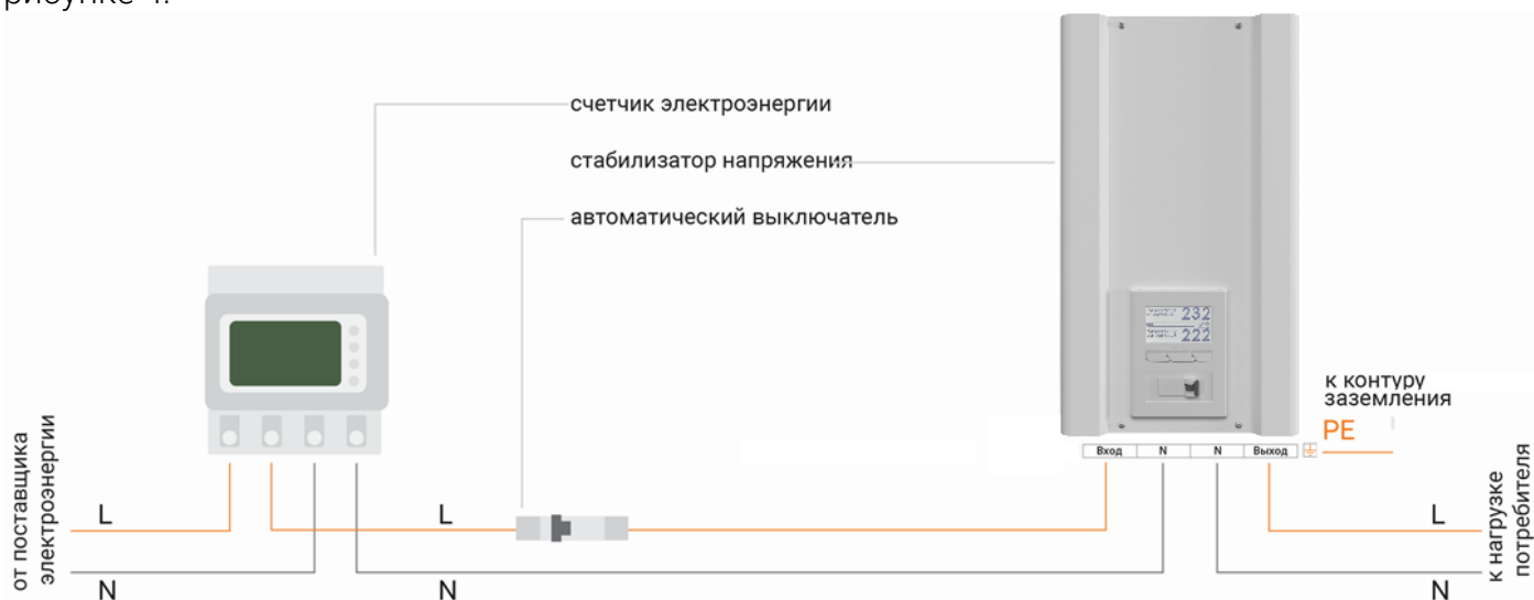
Рисунок 3. Схема подключения стабилизатора к однофазной сети
