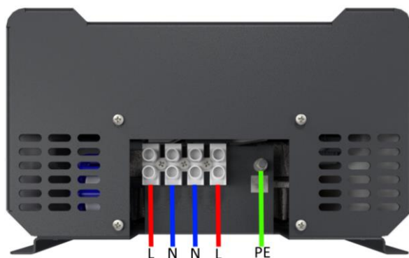
Рисунок 2. Схема подключения к клеммной колодке стабилизатора
