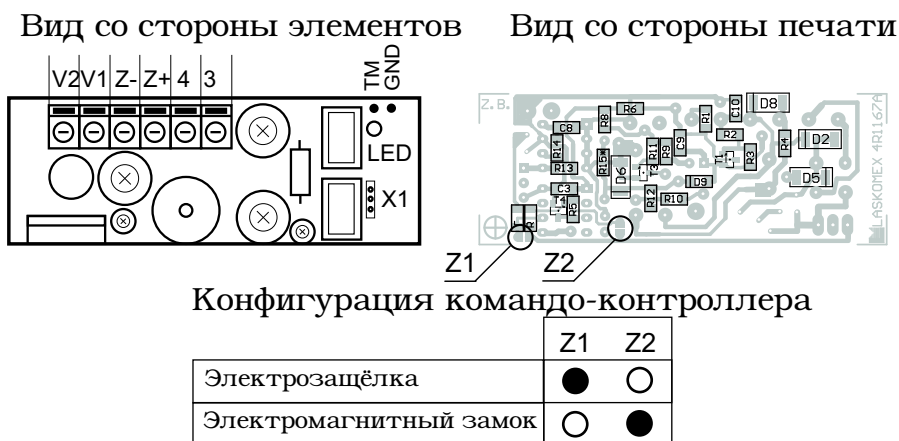
Рис. Вид платы считывателя ключей Dallas.
