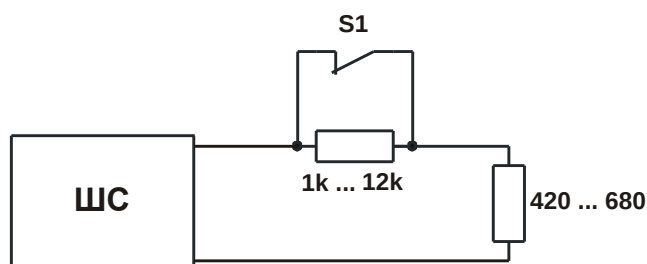
Рис. 6 Последовательное подключение 1-го извещателя с НЗ контактами.
