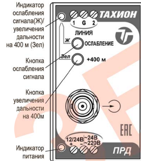
Рис.3 Передатчик
