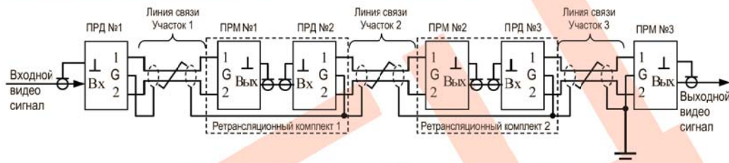
Рис.7 Схема построения линии связи с max длиной 4,8 км, при невозможности заземления на всех передающих сторонах
