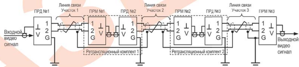
Рис.4. Схема построения линии с макс длиной 2100м с заземлением на всех передающих сторонах.
