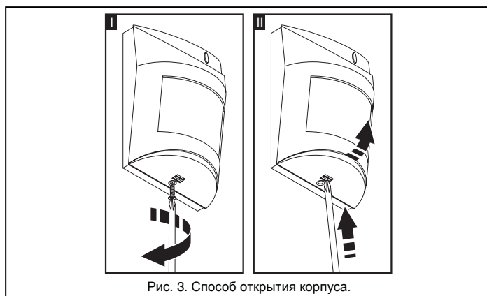
Рис. 3. Способ открытия корпуса.
