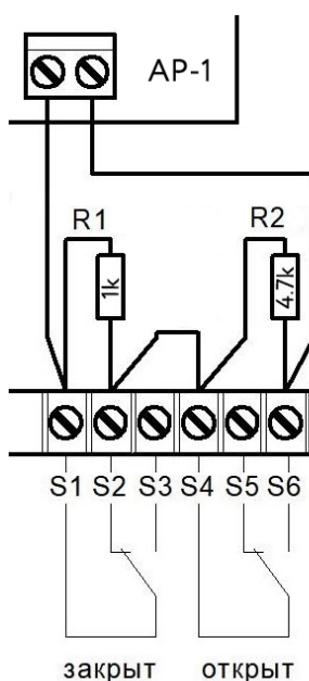
Рисунок 10 – Схема подключения
