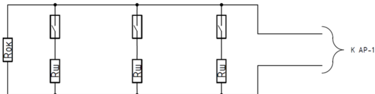
Рисунок 5 – Схема подключения бездресных устройств в нормальном состоянии NC
