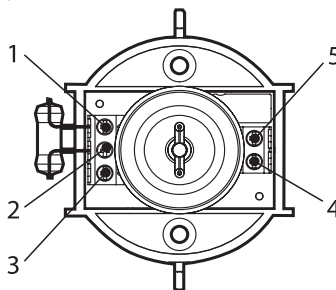
Рисунок 2. Клеммы извещателя.
