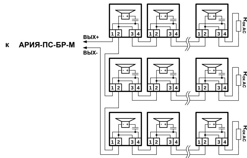
В. Схема соединений 6, 9, 12, 15, 18, 21, 24, 27, 30, 33 и 36-ти речевых оповещателей серии АРИЯ-ПС. Номинал оконечного резистора R_{ок\ AC} = 1,5\ k\Omega \pm 5\% .
