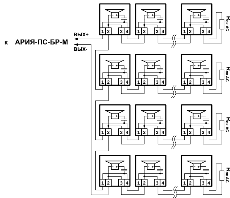
Г. Схема соединений 8, 12, 16, 20, 24, 28, 32, 36, 40, 44 и 48-ми речевых оповещателей серии АРИЯ-ПС. Номинал оконечного резистора R_{ок\ AC} Скачано с sec.ru
