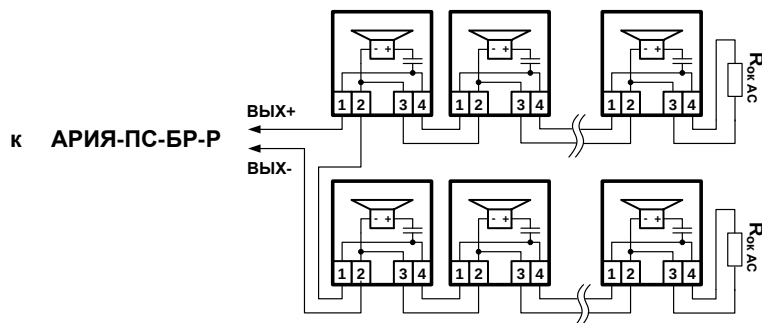
Б. Схема соединений 4, 6, 8, 10, 12, 14 и 16-ти речевых оповещателей серии АРИЯ-ПС. Номинал оконечного резистора R_{ок\ AC} = 2,4\ k\Omega \pm 5\% .
