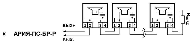
А. Схема соединений 1, 2, 3 и 4-х речевых оповещателей серии АРИЯ-ПС. Номинал оконечного резистора R_{ок\ AC} = 4,7\ k\Omega \pm 5\% .
