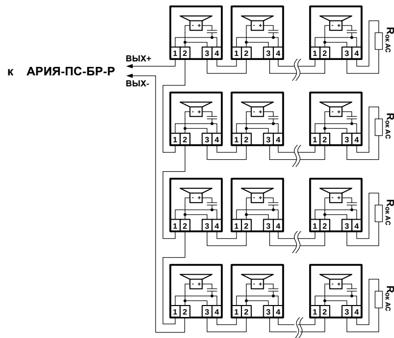
Г. Схема соединений 8, 12, 16, 20, 24, 28, 32, 36, 40, 44 и 48-ми речевых оповещателей серии АРИЯ-ПС. Номинал оконечного резистора R_{ок\ AC} = 1,5\ k\Omega \pm 5\% .
