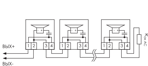
Рис. 17. Схема для 1, 2, 3 и 4 оповещателей. Номинал оконечного резистора R_{ок. АС} = 4,7 \text{ кОм} \pm 5\% .
