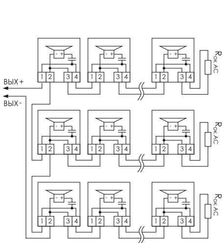
Рис. 17. Схема для 1, 2, 3 и 4 оповещателей. Номинал оконечного резистора R_{ок. АС} = 4,7 \text{ кОм} \pm 5\% .
