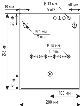
Рис. 61. Установочные размеры модификации АРИЯ-ПС-БРО-Р. Вид сзади
