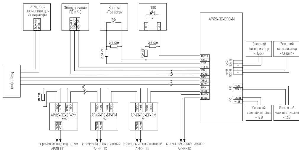
Рис. 10. Схема подключения оборудования к АРИЯ-ПС-БРО-М
