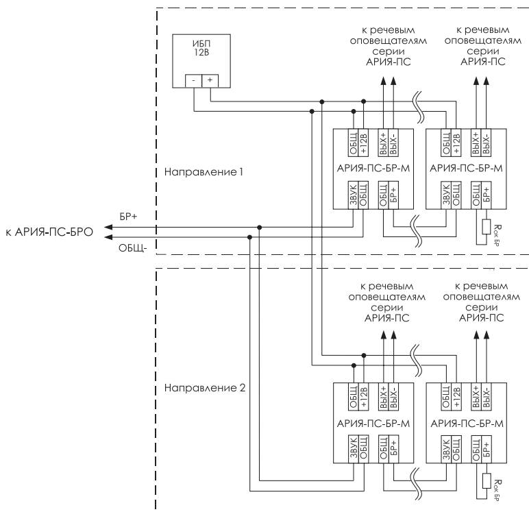
Рис. 15. Схема соединений для двух направлений линии управления. Номинал оконечного резистора R_{ок\ БР} = 10\ кОм \pm 5\ % .
