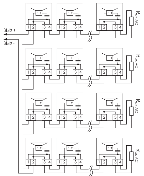
Рис. 20. Схема для 16, 20, 24, 28, 32, 36, 40, 44 и 48 оповещателей. Номинал окончного резистора R_{ок. АС} = 1,2 \text{ кОм} \pm 5\% .
