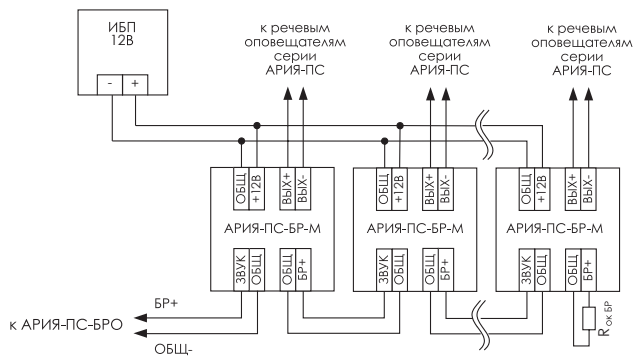
Рис. 14. Схема соединений для одного направления линии управления. Номинал оконечного резистора R_{ок\ БР} = 4,7\ кОм \pm 5\ % .
