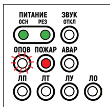
Рис. 44. Индикация при отсчете времени задержки воспроизведения речевого сообщения
