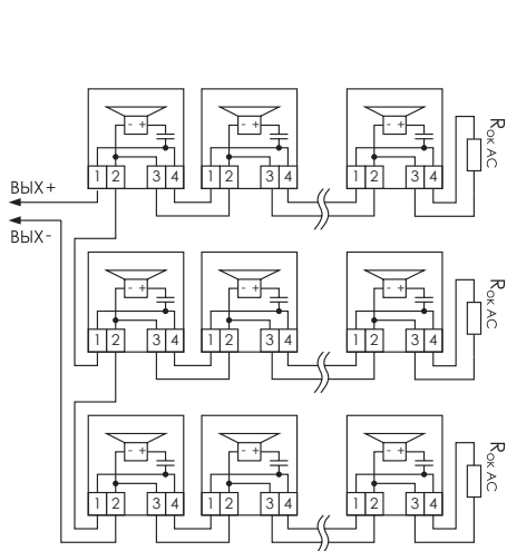
Рис. 17. Схема для 1, 2, 3 и 4 оповещателей. Номинал оконечного резистора R_{ок AC} = 4,7 \text{ кОм} \pm 5\% .
