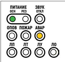
Рис. 50. Индикация при отключении напряжения питания от резервного источника
