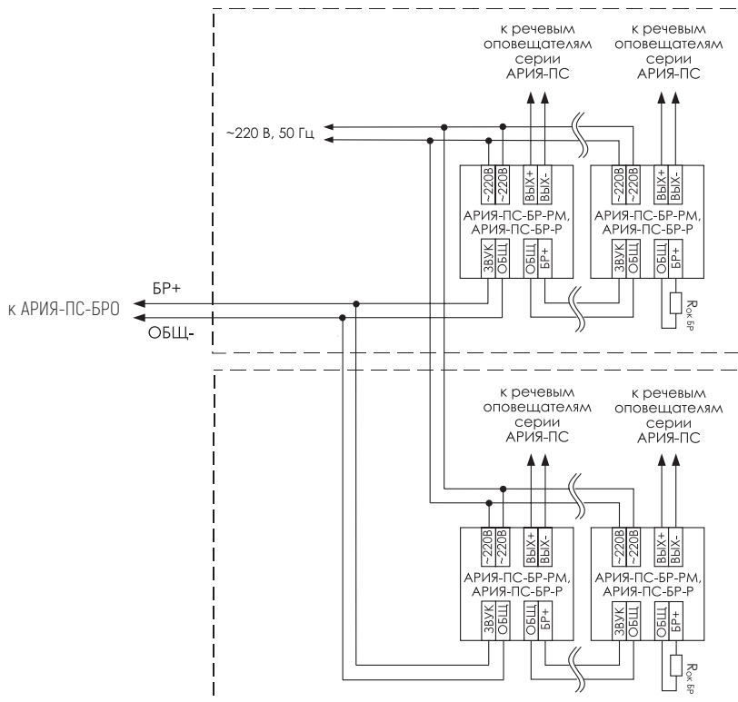
Рис. 12. Схема соединений для двух направлений линии управления. Номинал оконечного резистора R_{ок} БР = 10 кОм \pm 5\% .
