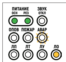
Рис. 59. Индикация после устранения неисправности
