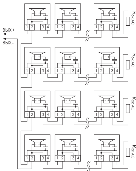
Рис. 20. Схема для 16, 20, 24, 28, 32, 36, 40, 44 и 48 оповещателей. Номинал оконечного резистора R_{ок AC} = 1,2 \text{ кОм} \pm 5\% .
