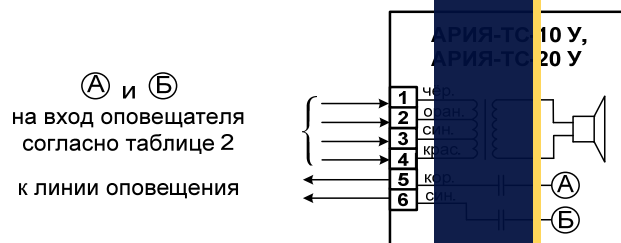
Рис.1. Схема подключения.
