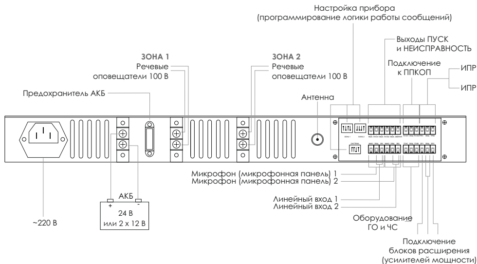
Рис. 7. Задняя панель АРИЯ-ТС-БРО-РМ-2-120
