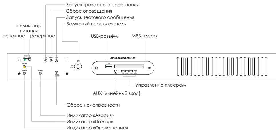
Рис. 4. Передняя панель АРИЯ-ТС-БРО-РМ-120
