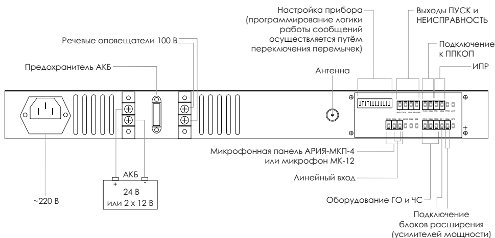
Рис. 5. Задняя панель АРИЯ-ТС-БРО-РМ-120
