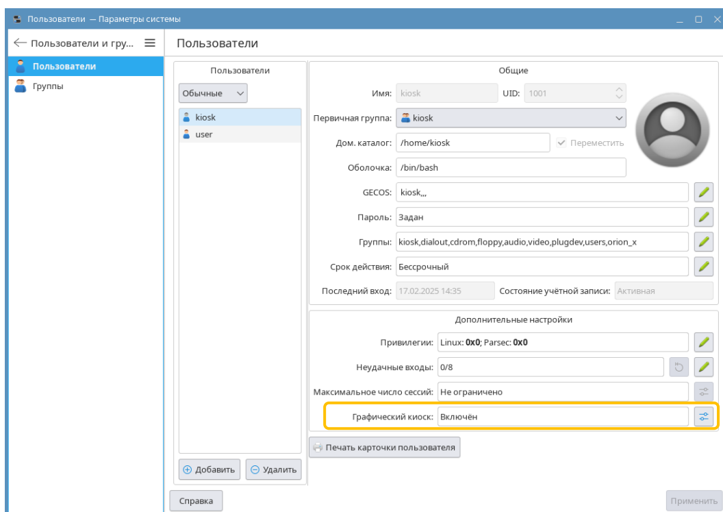
Рисунок 14 – Окно «Пользователи» с указанием о включённом режиме графический киоск
