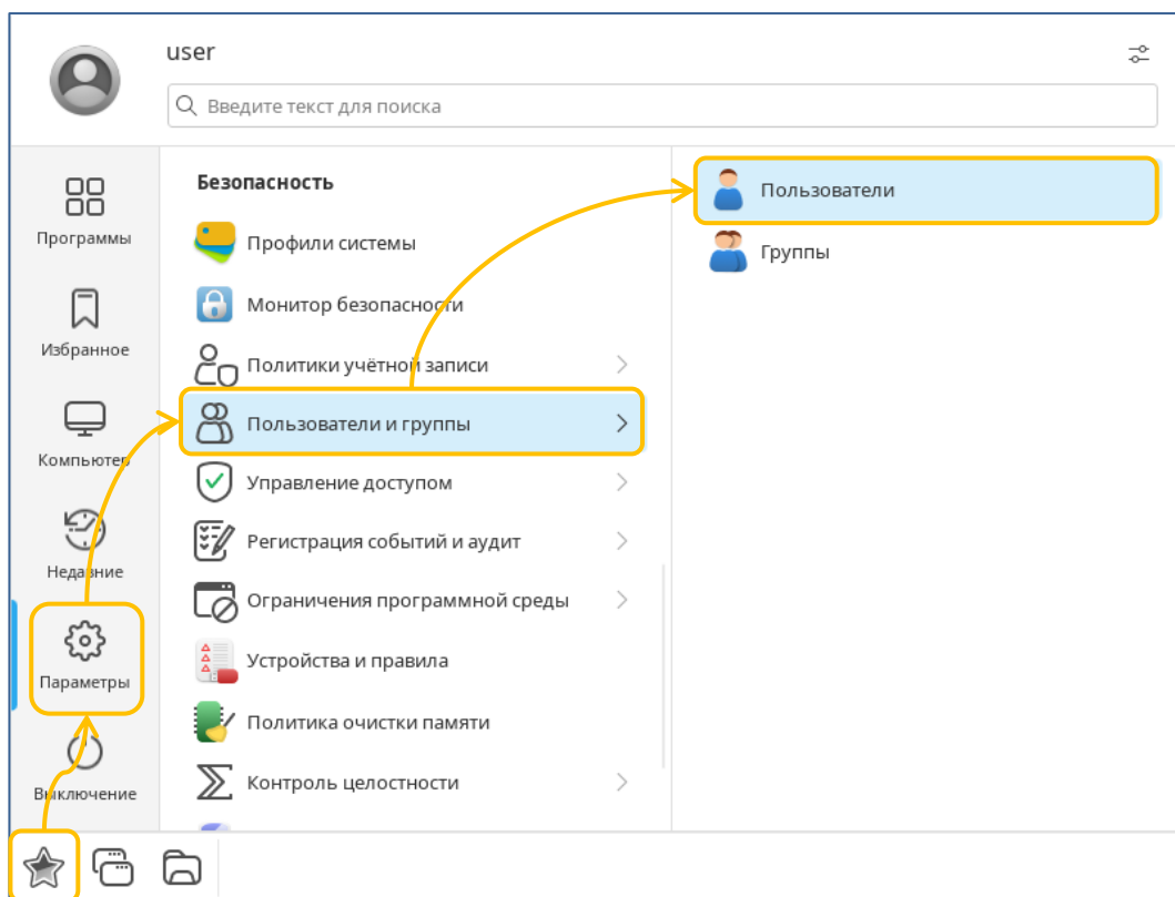
Рисунок 5 – Путь открытия окна «Пользователи»
