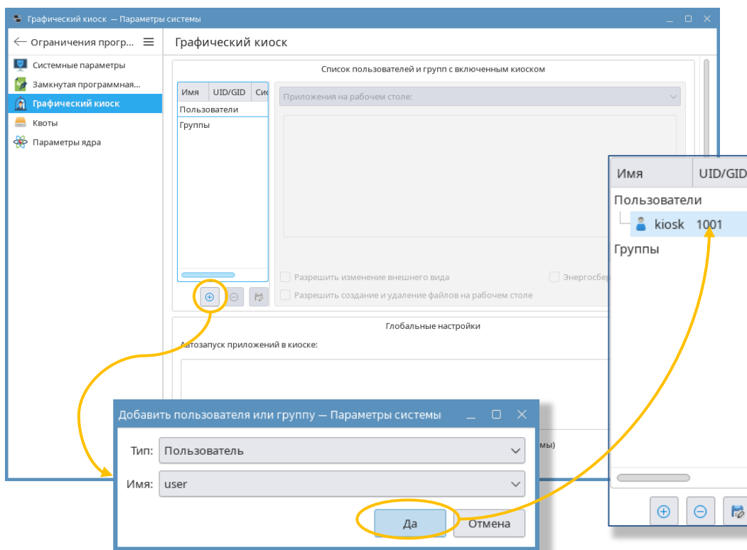
Рисунок 11 – Окно «Графический киоск» и настройка пользователя
