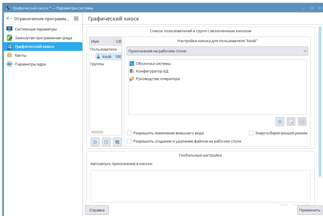
Рисунок 13 – Пример настроенного режима графический киоск
