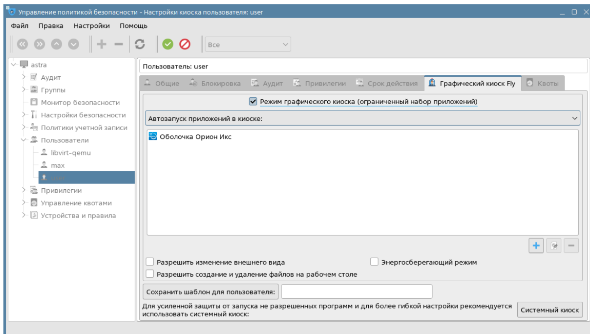
Рисунок 16 – Настройка автозапуска АРМ «Орион Икс»
