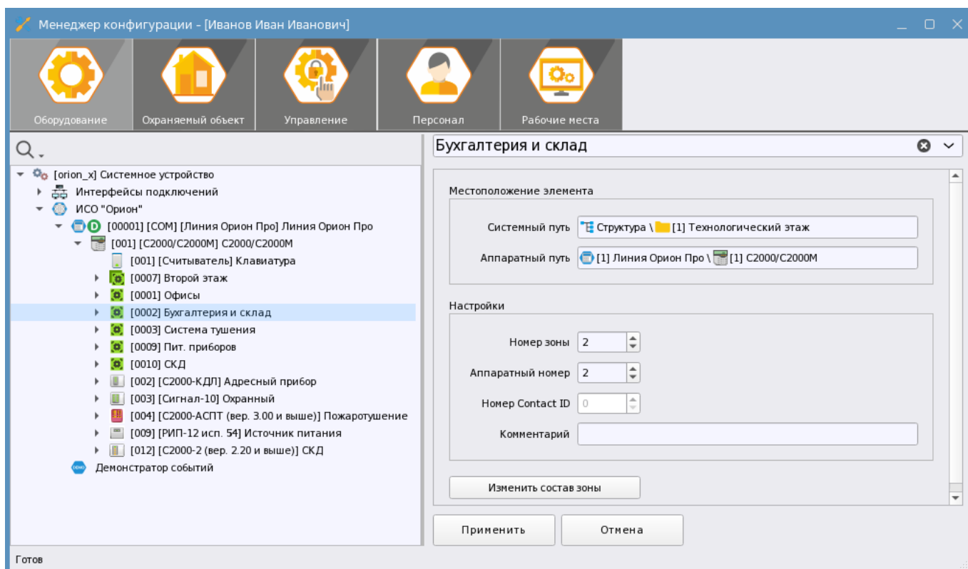
Рисунок 79 – Вкладка «Оборудование»
