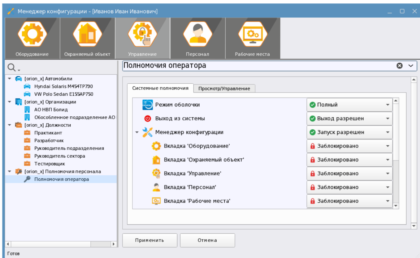
Рисунок 217 – Вкладка «Управление»
