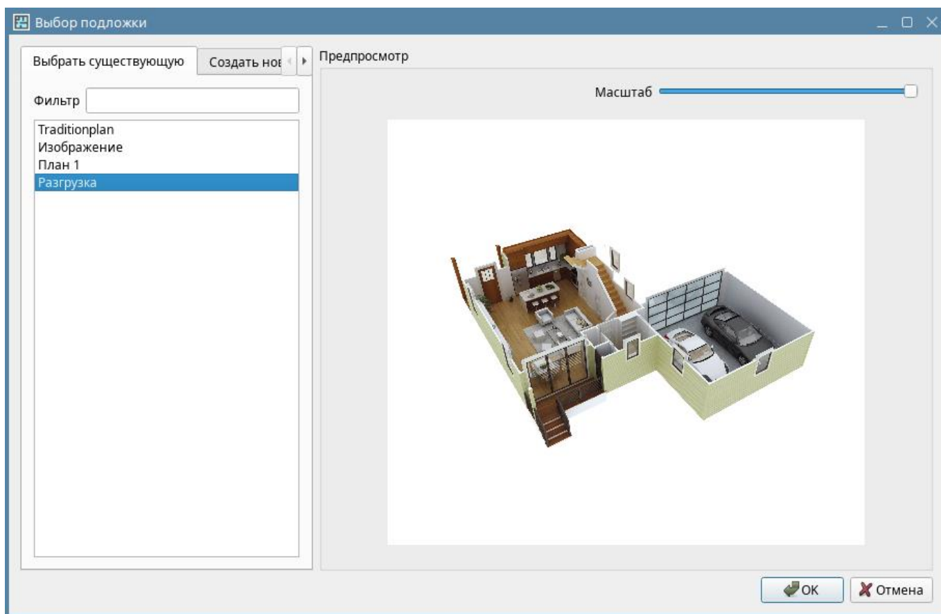
Рисунок 190 – Выбор подложки
