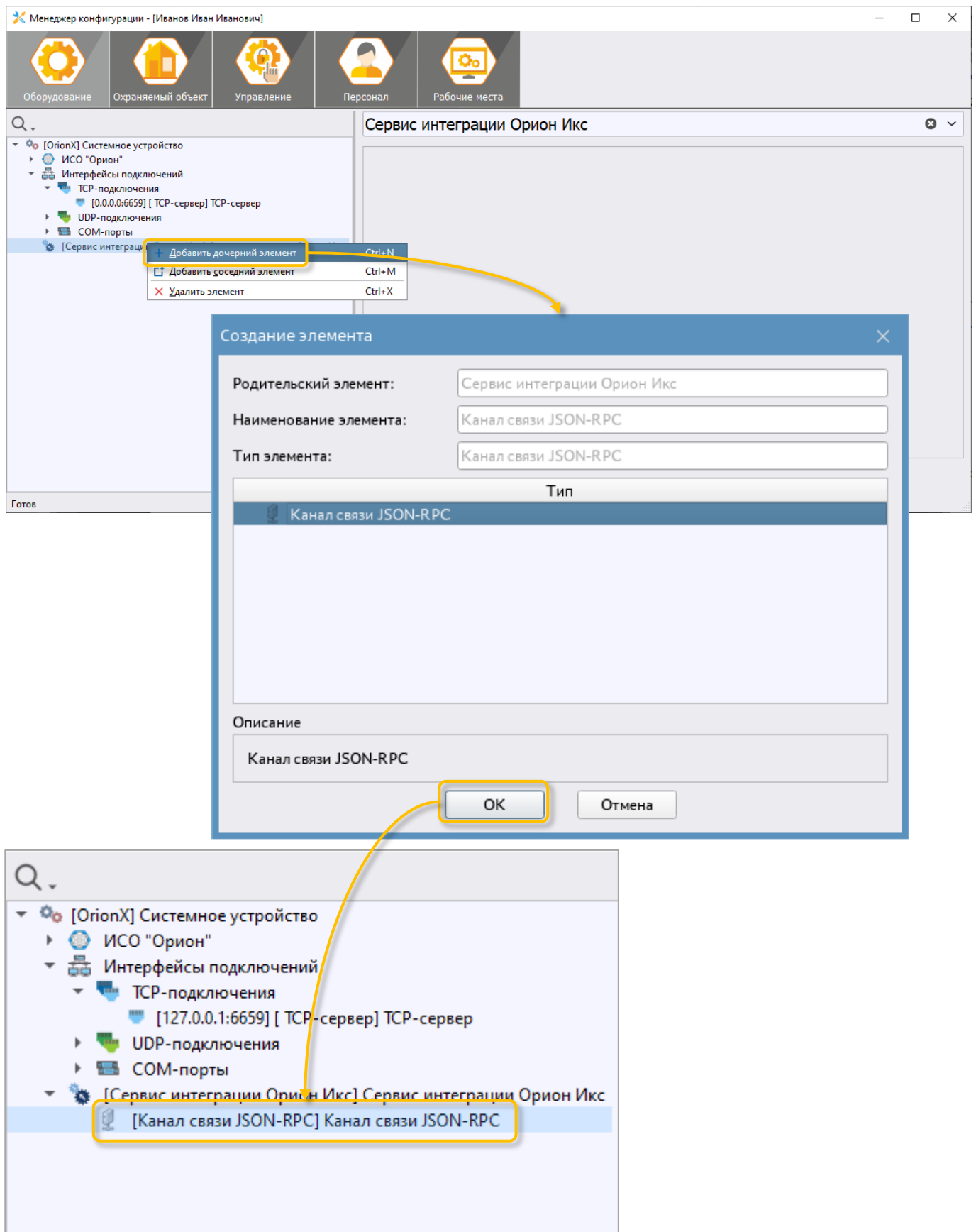
Рисунок 4 – Подключение канала связи JSON-RPC
