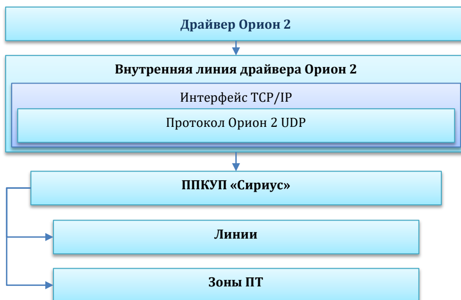
Рис. 4-1 Схематическое отображение структуры подключения к драйверу Орион 2
