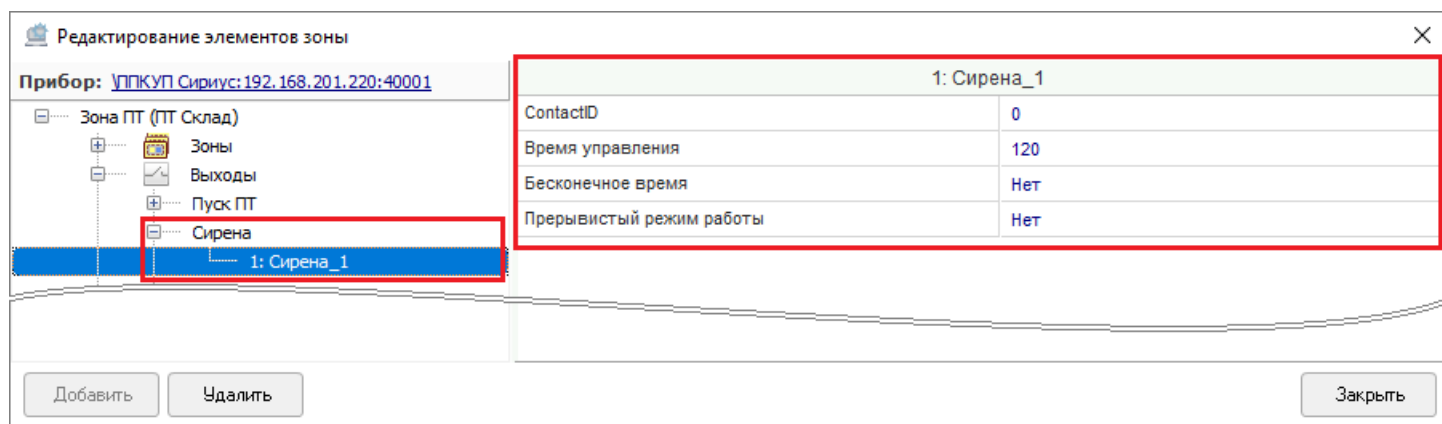
Рис. 4-14 Параметры выхода "Сирена"
