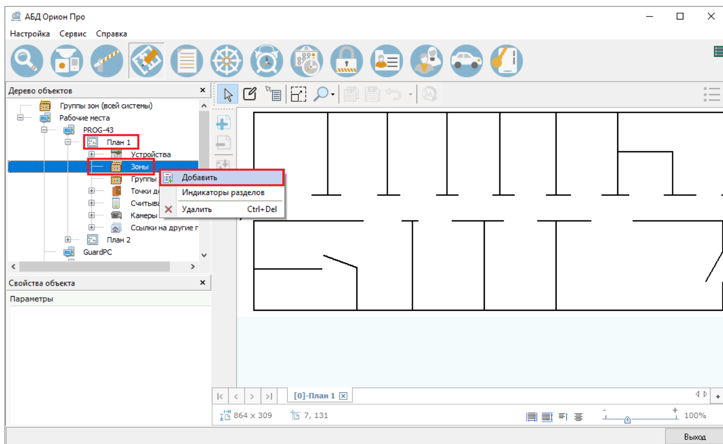
Рис. 4-32 Добавление зоны ПТ в соответствующий узел плана помещений
