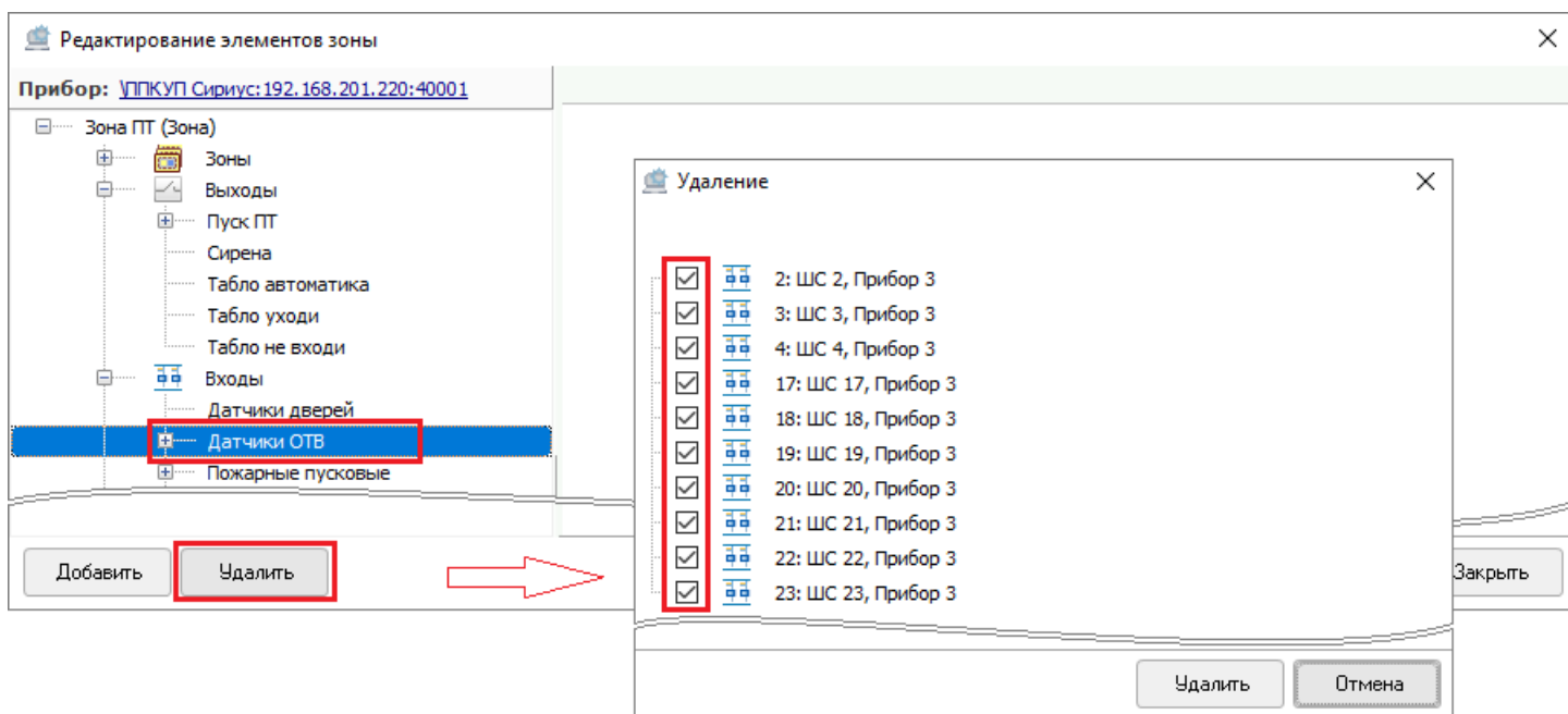
Рис. 4-25 Удаление датчиков ОТВ способом массового выделения всех элементов узла
