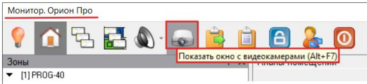
Рисунок 5.7 – Монитор ОЗ
