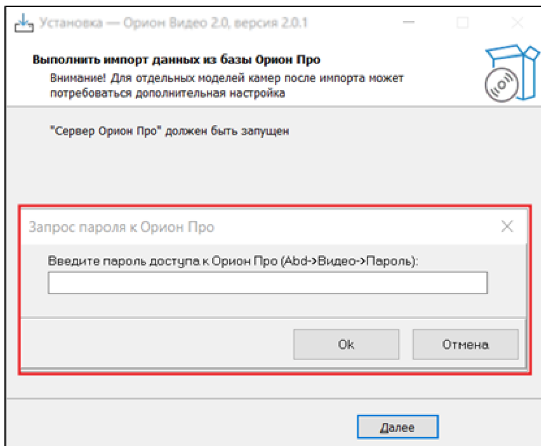
Рисунок 5.13 – Запрос импорта
