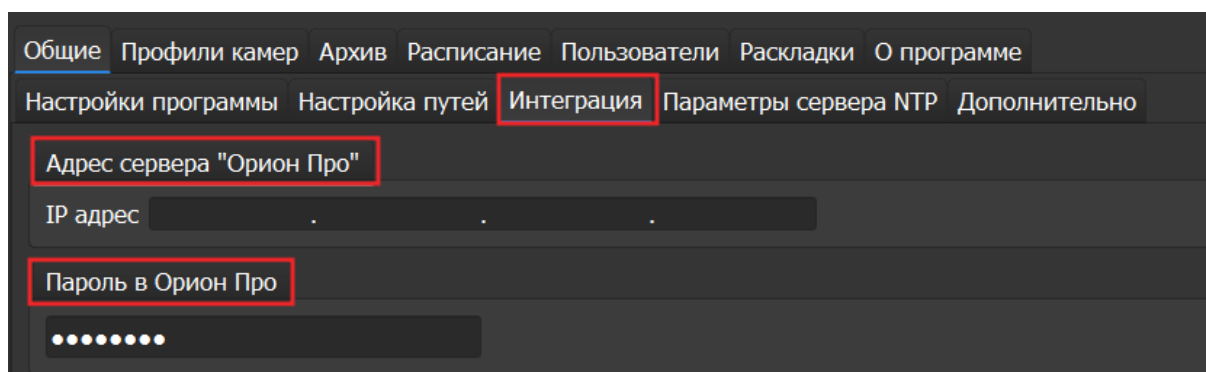
Рисунок 5.11 – Интеграция
