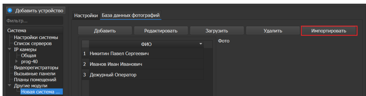
Рисунок 5.9 – Импорт
