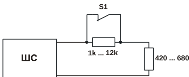
Рис. 4 Последовательное подключение 1 извещателя с НЗ контактами.
