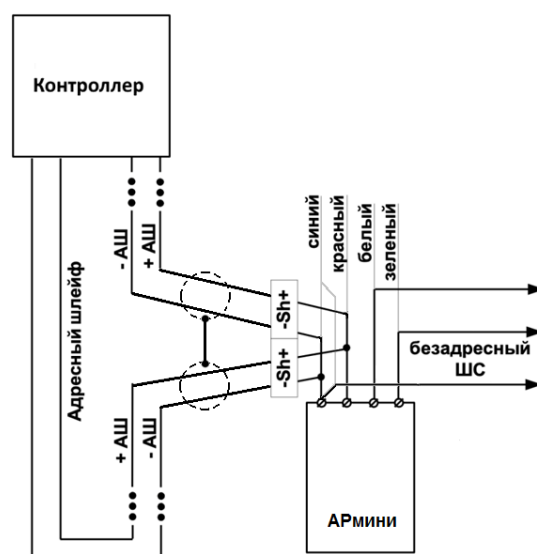
Рис. 2 Подключение АРмини исп.09 с одним безадресным ШС
