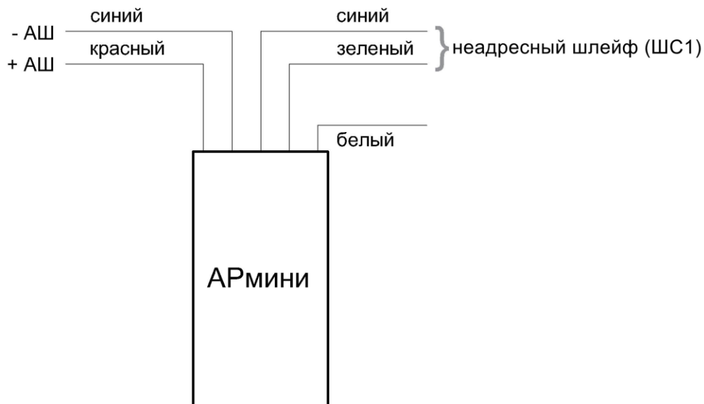
Рис. 8 Подключение к АРмини исп.09 одного неадресного ШС
