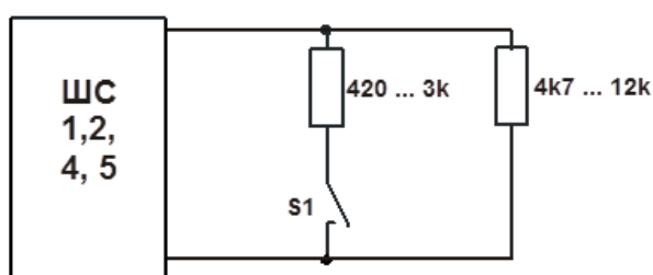
Рис. 5 Параллельное подключение 1 извещателя с НР контактами.
