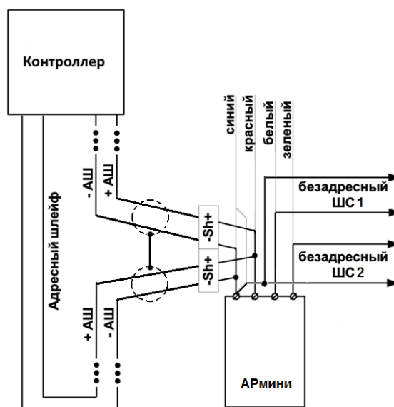
Рис. 3 Подключение АРмини исп.09 с двумя безадресными ШС
