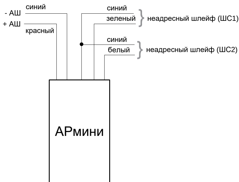
Рис. 9 Подключение к АРмини исп.09 двух неадресных ШС
