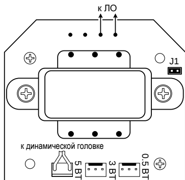
Рис.1 Плата АС
