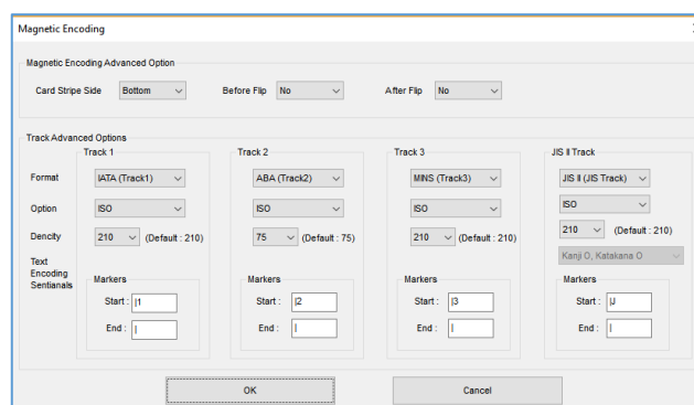
Рис. 38 Настройка опций кодировки магнитной полосы
