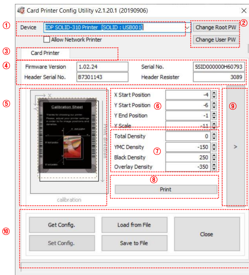
Рис. 48 CardPrinterConfig – Базовые установки Принтера карт
