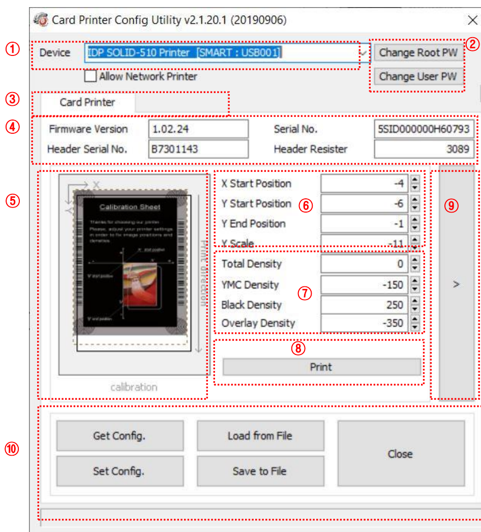
Рис. 64 CardPrinterConfig – Базовые установки Принтера карт
