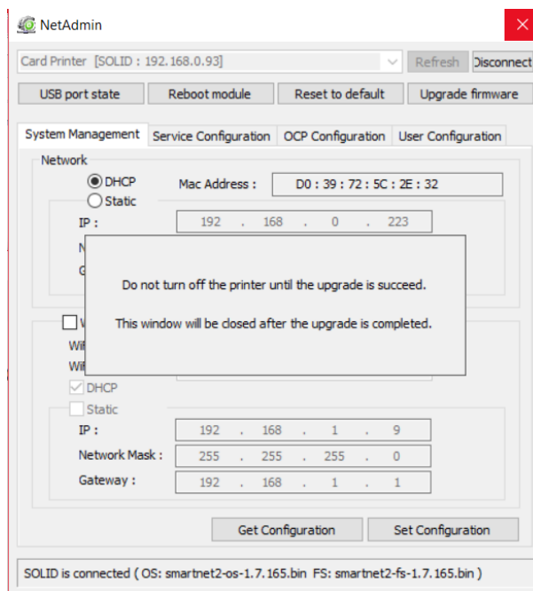
Рис. 82 Обновление прошивки (Firmware)
