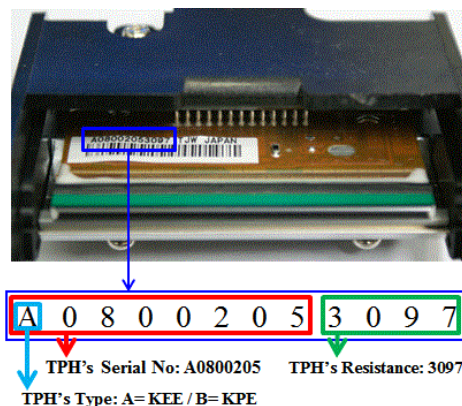
Рис. 111 Термопечатная головка
