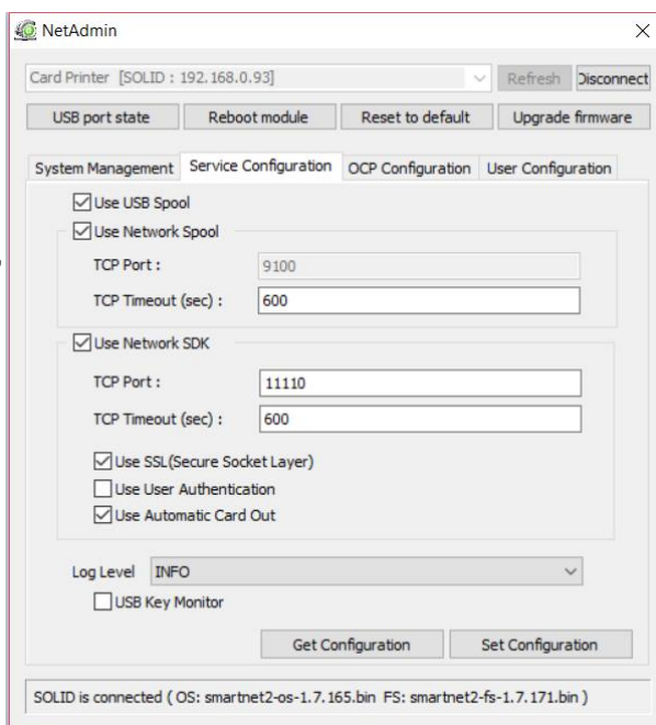
Рис. 86 Сетевое сервисное конфигурирование
