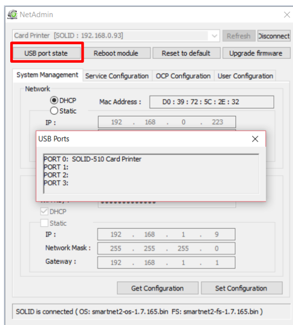
Рис 78 Состояние USB порта
