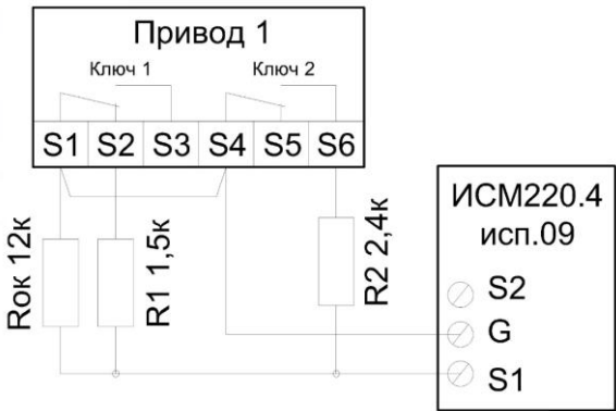
Подключение концевиков
