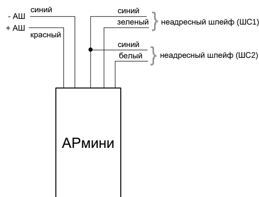
Подключение двух неадресных ШС
