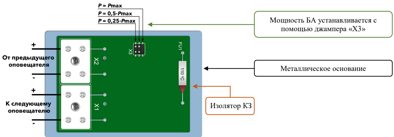
Рисунок 3. Схема подключения и установки мощности БА АСР-01.1.8 исп. XX.ЕА с двумя керамическими клеммными колодками на металлическом основании, с изолятором КЗ, с возможностью контроля по переменному току (импедансу).
