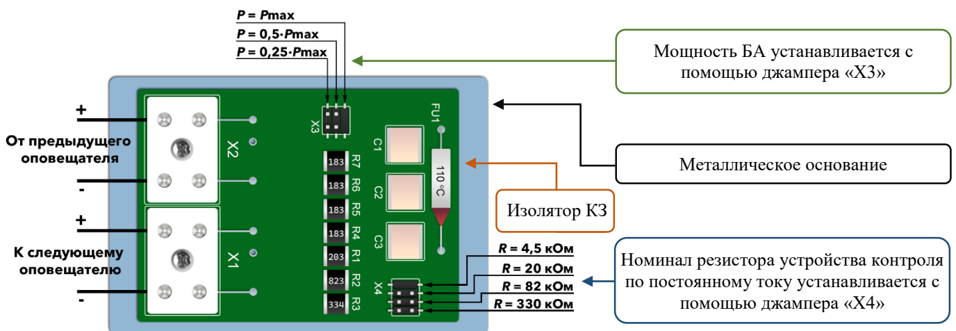
Рисунок 4. Схема подключения и установки мощности БА АСР-01.1.8 исп. XX.МА с двумя керамическими клеммными колодками на металлическом основании, с изолятором КЗ, с устройством контроля по постоянному току.
