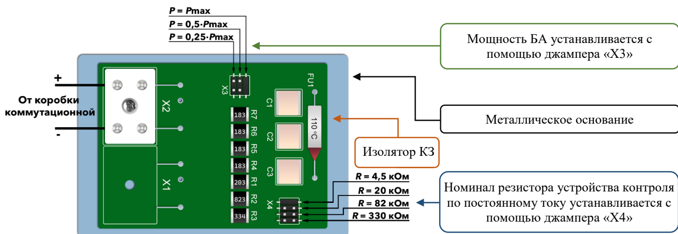
Рисунок 5. Схема подключения и установки мощности БА АСР-01.1.8 исп. XX.НА с одной керамической клеммной колодкой на металлическом основании, с изолятором К3, с устройством контроля по постоянному току.
