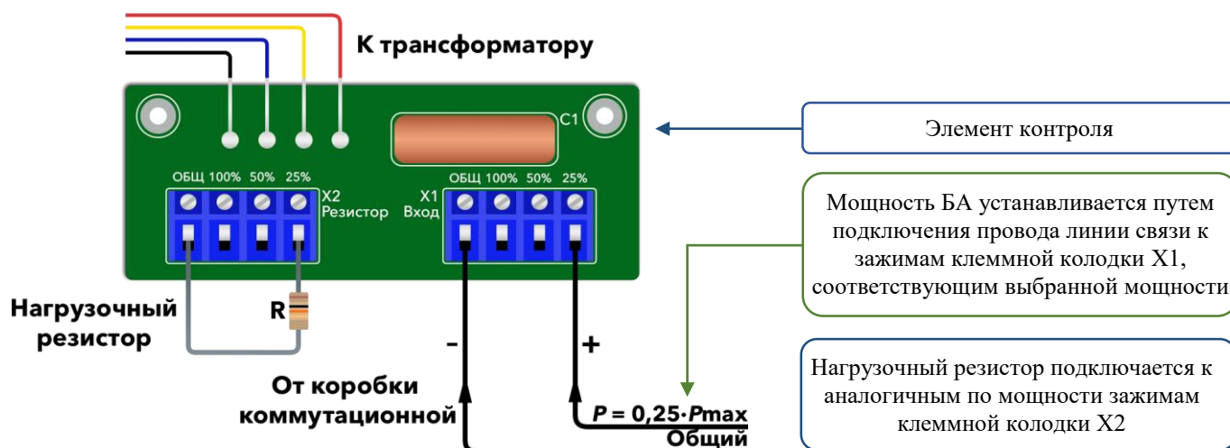
Рисунок 6.3. Схема подключения и установки мощности P_{\text{max}} = 0,25 Вт БА АСР-01.1.8 исп. XX.КА с пластиковыми клеммными колодками, с элементом контроля по постоянному току.
