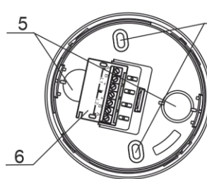
База с платой изолятора короткого замыкания Электронный блок снят
