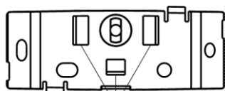
Пазы для установки кронштейна Астра-5/621
