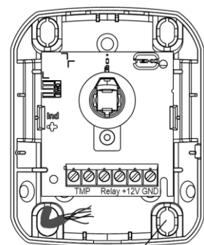
Заглушка отверстия для проводов
