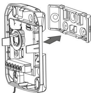
Заглушка отверстия для проводов
