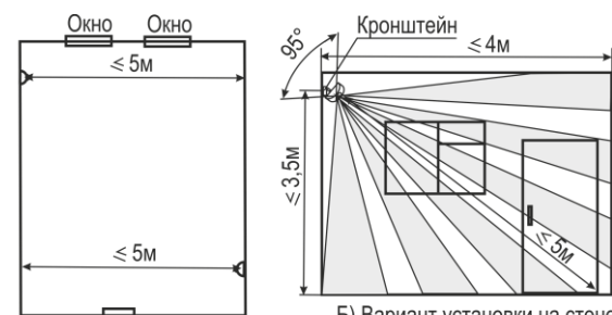
А) Вариант установки на стене (вид сверху)
