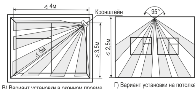
В) Вариант установки в оконном проеме
