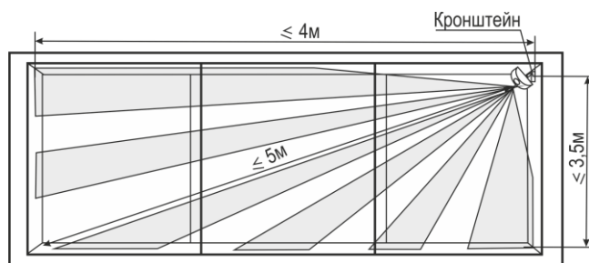
Д) Вариант установки между рамами
