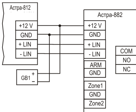
Рисунок 7 - Схема подключения ППКОП «Астра-812» в расширенном режиме работы коммутатора
