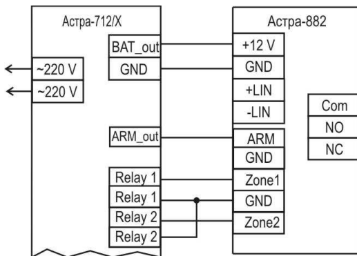
Рисунок 4 - Схема подключения ППКОП «Астра-712/Х» в автономном режиме работы коммуникатора
