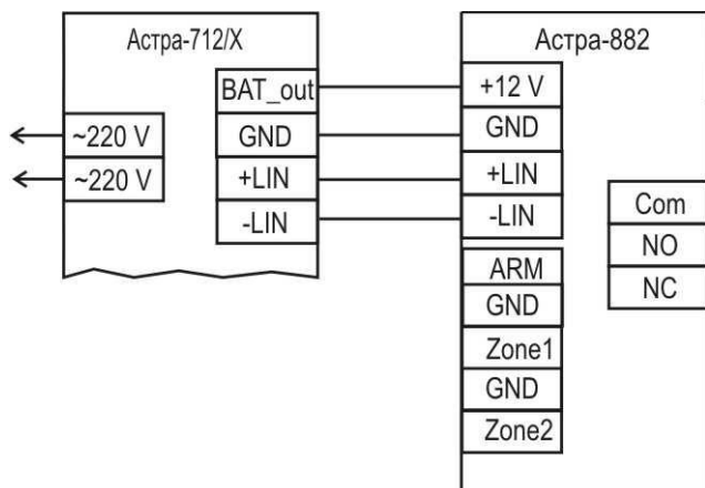
Рисунок 6 - Схема подключения ППКОП «Астра-712/X» в расширенном режиме работы коммуникатора
