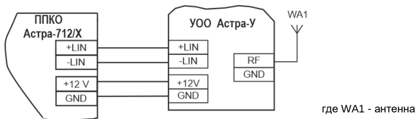
Рисунок 7 - Схема подключения ППКО
