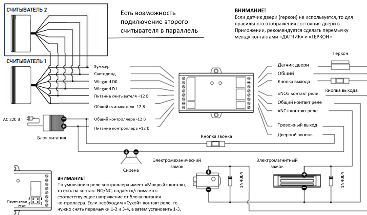
Схема подключения контроллера *****
