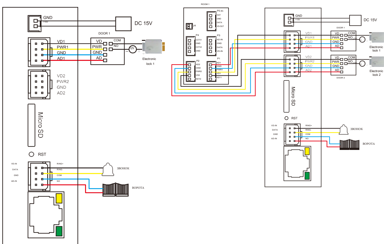
Схема 4. Подключение WI-FI Вых к вызывной панели.
