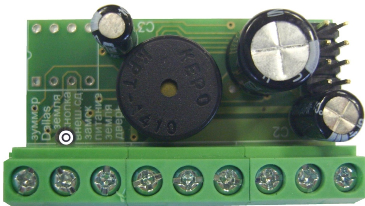
Рис.1 Внешний вид платы контроллера
