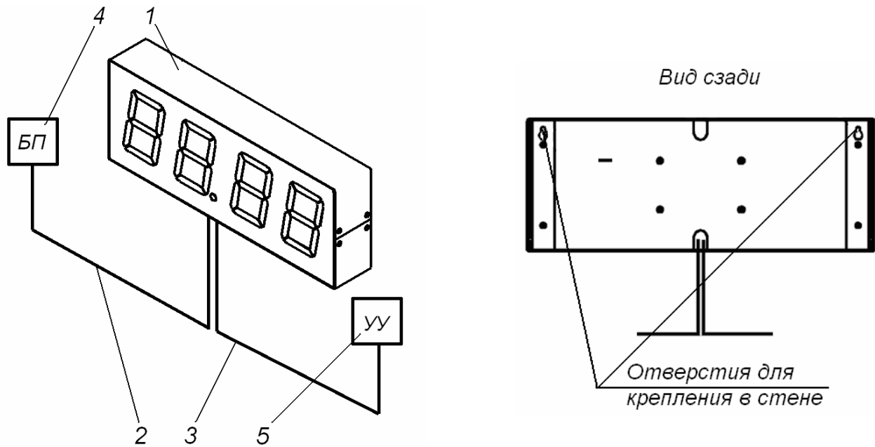
Рисунок 1. Устройство ТСВ:
