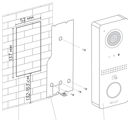
Монтажная обложка Кронштейн Вызывная панель
