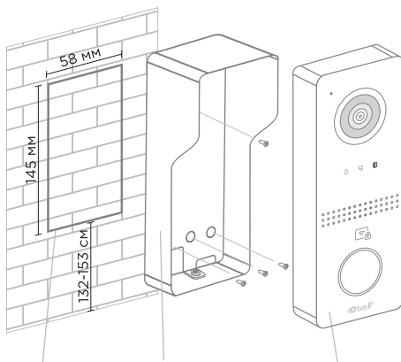
Монтажная обложка Кронштейн Защита от солнца и дождя Вызывная панель
