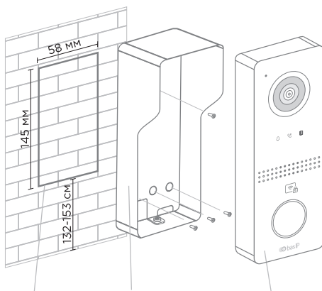
Монтажная обложка Кронштейн Вызывная панель
