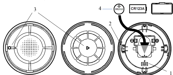
1 – Кнопка "ПРОГ" для инициализации устройства; 2 – Датчик снятия с базового основания; 3 – Светодиодный индикатор; 4 – Основная и резервная батареи
