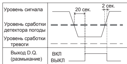
Проводное подключение погодного датчика отдельным шлейфом (схема Н.3.)
