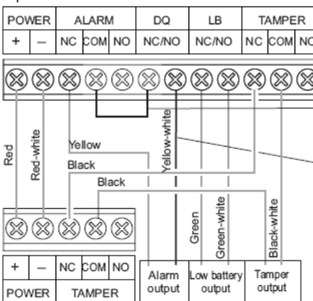
Подключение датчика погоды одним шлейфом вместе с тревожным выходом (схема Н.3.)
