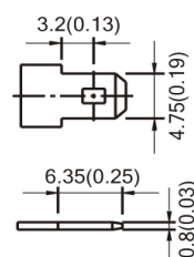
Вывод T1
