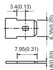
Вывод T2
