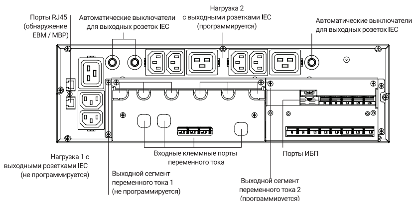
Вид сзади
