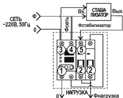
Рисунок 2 – Схема подключения.
