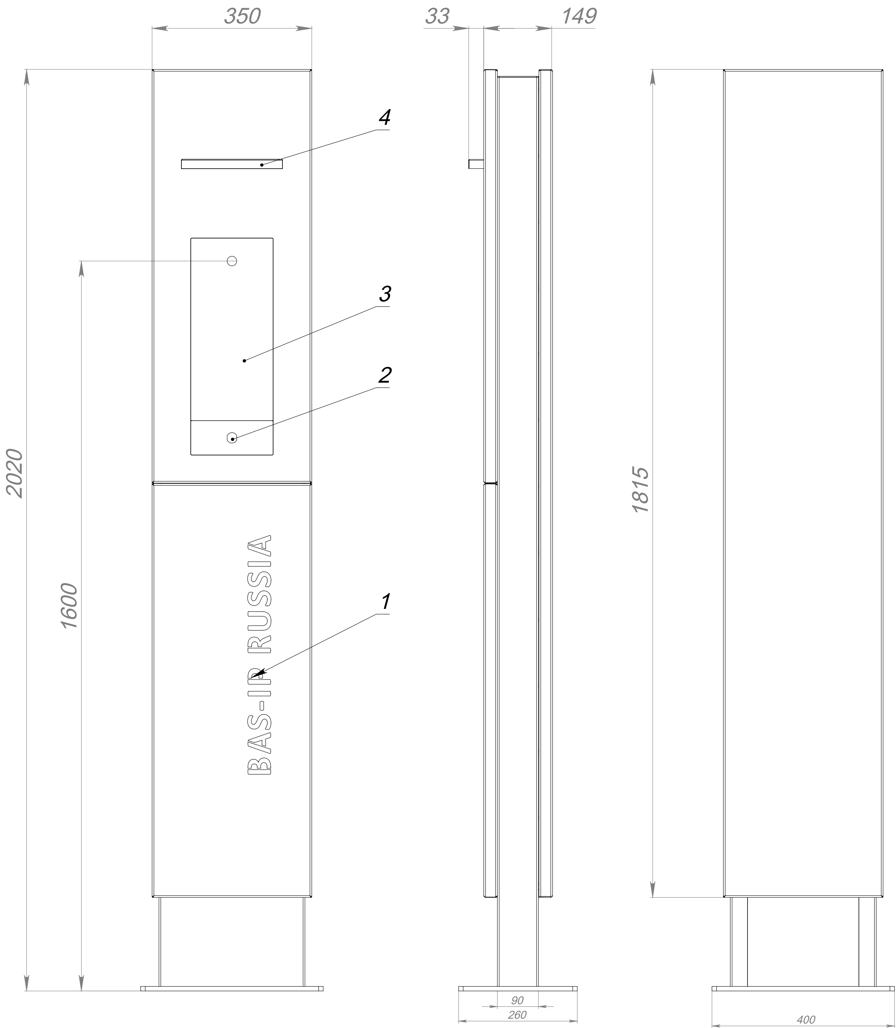
Рис.1 Внешний вид, габаритные размеры
