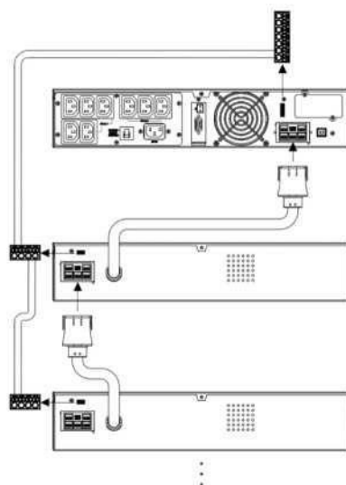
Рис. 3. Пример подключения внешнего батарейного блока к ИБП
