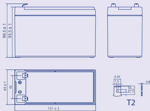
РАЗМЕРЫ | Клемма T2 (размеры в мм)
