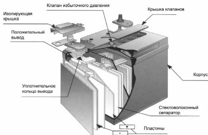
Рис. 1. Основные элементы конструкции аккумулятора технологии AGM с клапаном избыточного давления.
