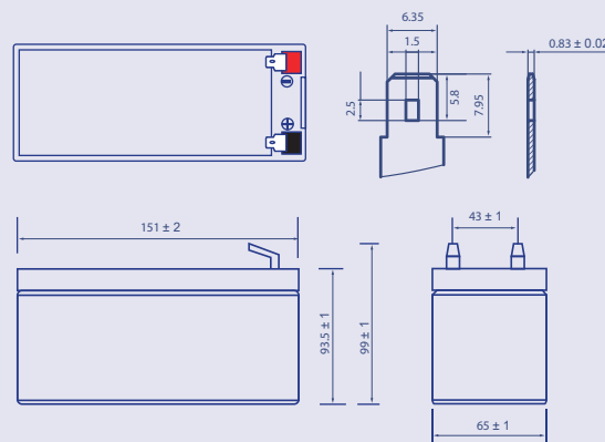
РАЗМЕРЫ | Клемма T1 (размеры в мм)
