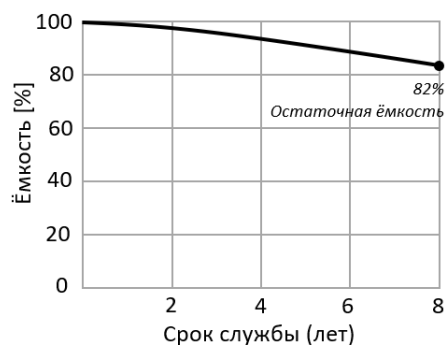
Рис. 2. Зависимость ёмкости АБ от срока службы для моделей ЛКД-АКБ-М со сроком службы до 8 лет. Модели: ЛКД-АКБ-12012-М, ЛКД-АКБ-12022-М, ЛКД-АКБ-1205-М, ЛКД-АКБ-1207-М, ЛКД-АКБ-1209-М, ЛКД-АКБ-1212-М, ЛКД-АКБ-1217-М, ЛКД-АКБ-1226-М.
