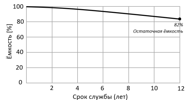
Рис. 3. Зависимость ёмкости АБ от срока службы для моделей ЛКД-АКБ-М со сроком службы до 12 лет. Модели: ЛКД-АКБ-1233-М, ЛКД-АКБ-1240-М, ЛКД-АКБ-1255-М, ЛКД-АКБ-1265-М, ЛКД-АКБ-12100-М, ЛКД-АКБ-12120-М, ЛКД-АКБ-12150-М, ЛКД-АКБ-12200-М.
