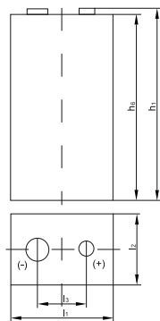
Рисунок 2 – Габаритные размеры 6LR61
