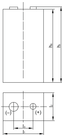
Рисунок 2 – Габаритные размеры 6LR61
